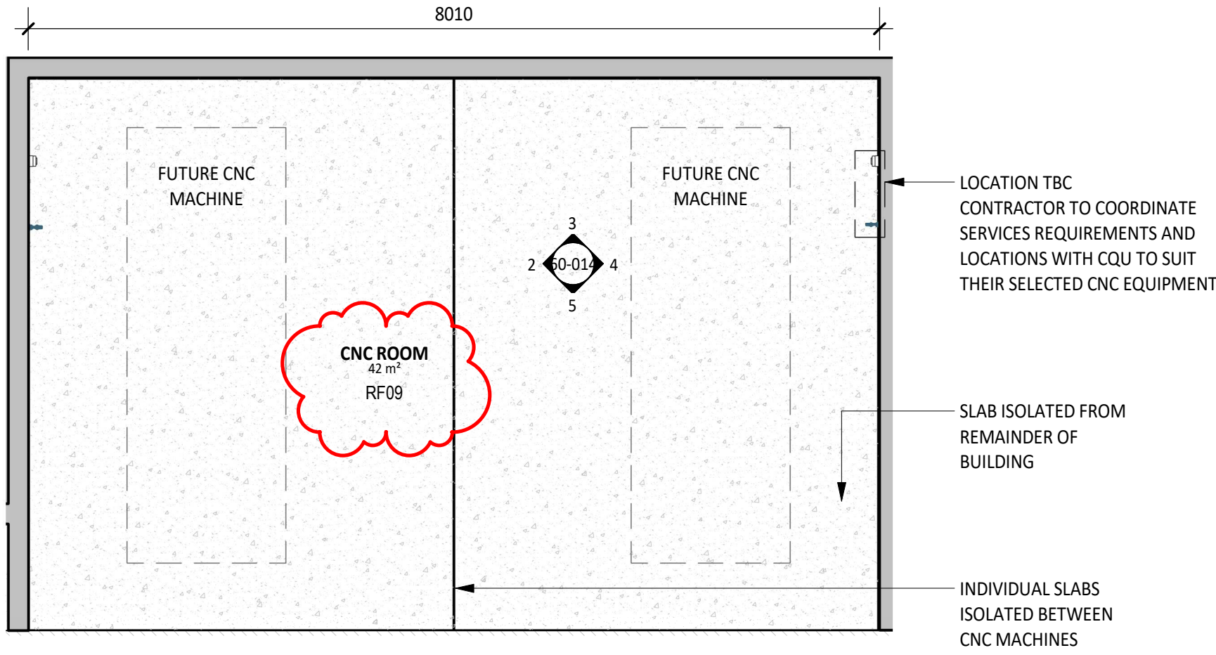
1 PLAN DETAIL 30-01 1 : 50
